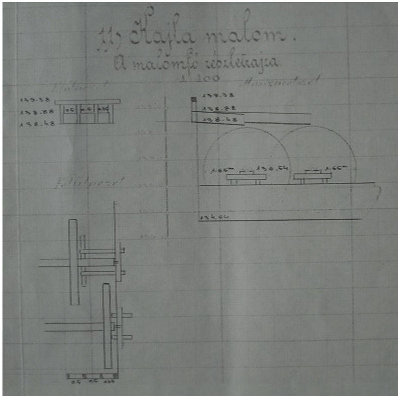
Kajla malom, a malomfő részletrajza a két vízkerékkal
