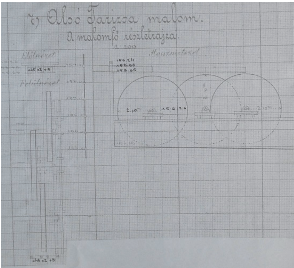
Az Alsó Tarizsa malom részletrajza 3 vízikerekkel
